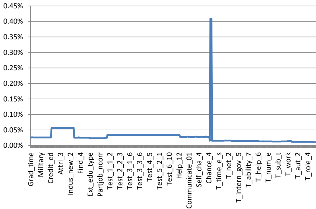
圖 2 各題項遺漏值分析
