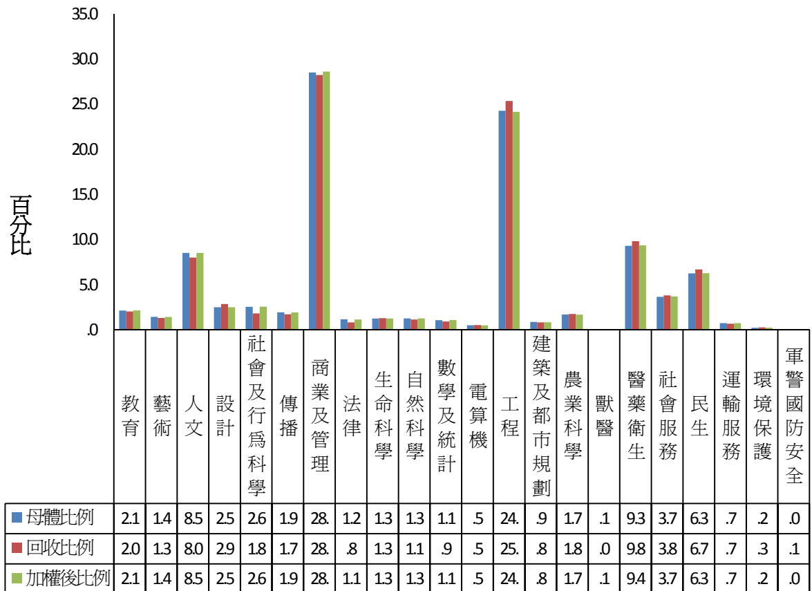
圖 1 各學門回收權重調整比較圖
